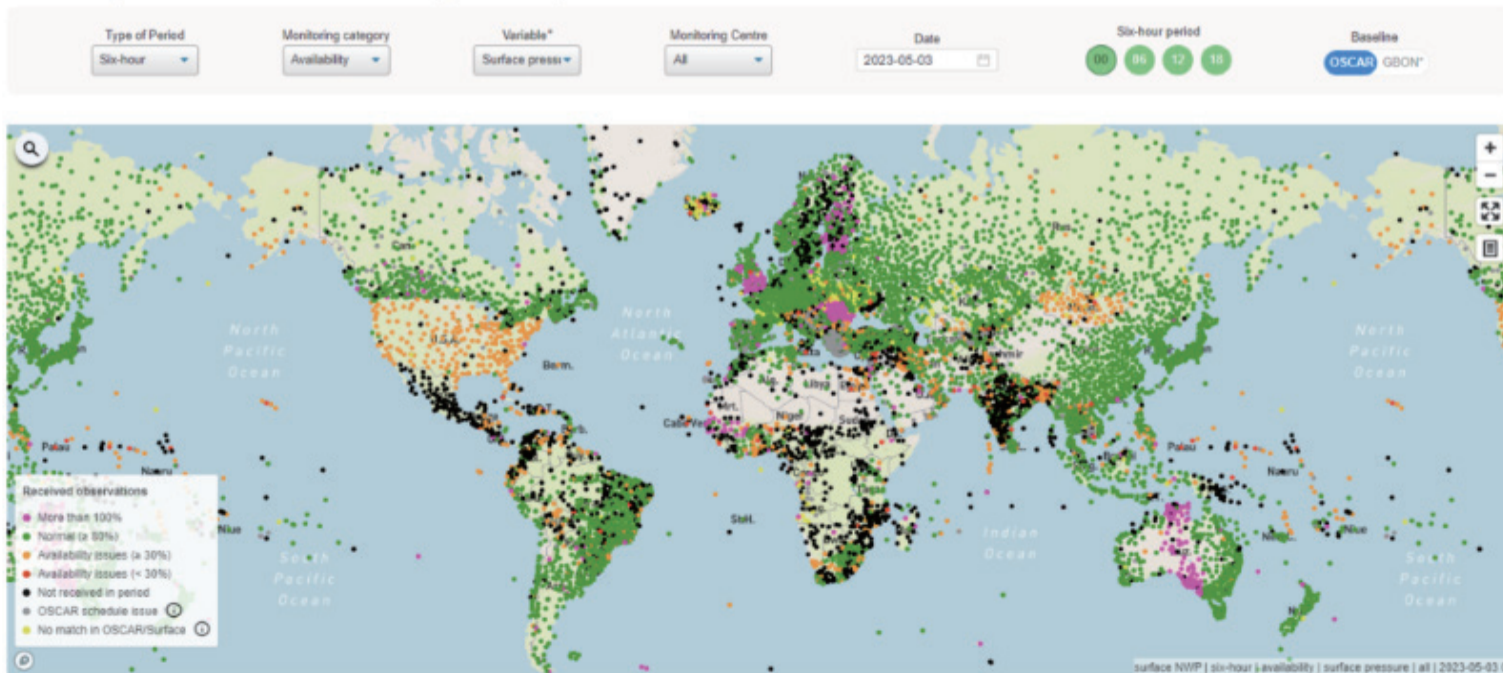
世界气象组织全球气候观测图网，红色代表观测密度最高 图片来源：丽塔教授
