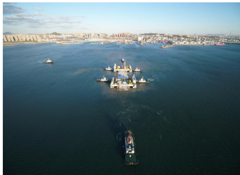
大连湾海底隧道施工资料图。(受访者供图)
