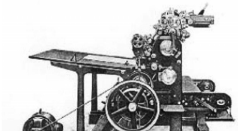
承印了《苏加诺总统藏画集》的国产第一代胶印机——老式安利机
